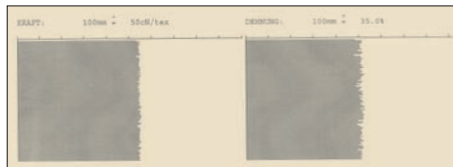
Viscose SULKY® en test de force-allongement: bonne solidité à la rupture totale
